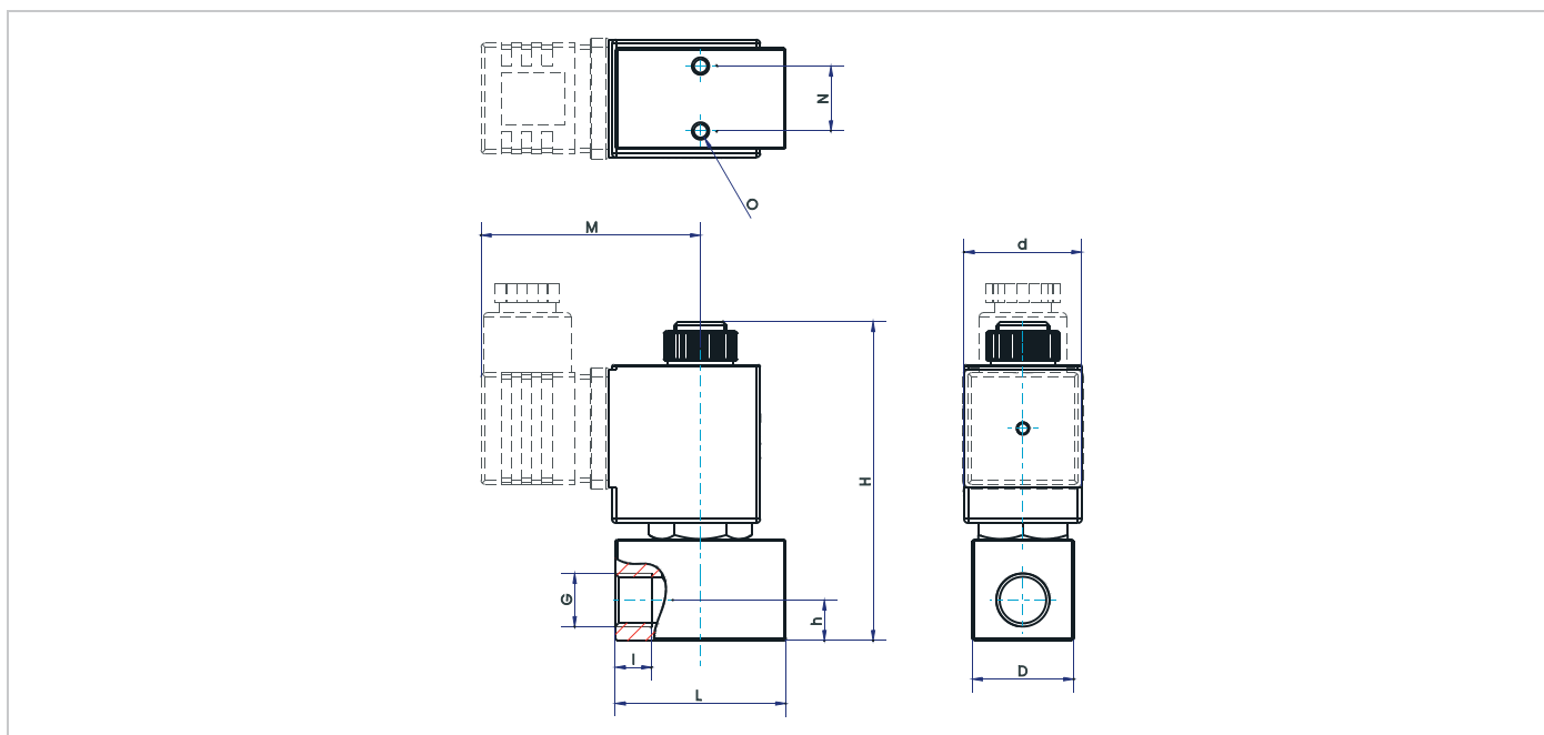
Maßtabelle für Typ 20 in mm, Gewicht ca. in g
